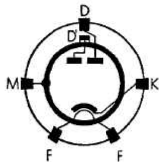
Sockelschaltung
